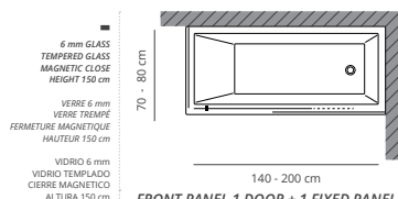
FRONT PANEL 1 DOOR + 1 FIXED PANEL PANNEAU FRONTAL PORTE + 1 PANNEAU FIXE PANEL FRONTAL 1 PUERTA + 1 PANEL FIJO
